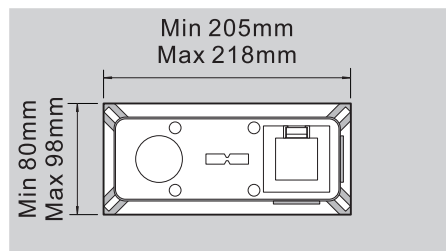
封牆後維修孔尺寸
