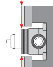
磁磚完成面 要切齊預埋盒上緣
